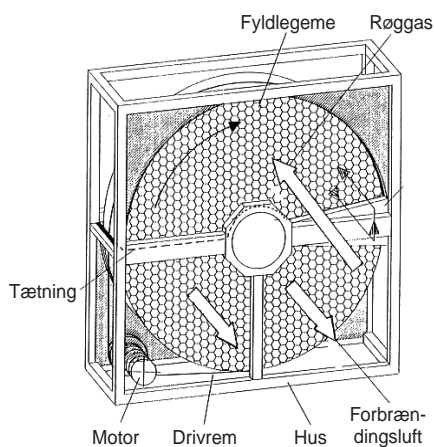
Figur 1. Principet i optinox-rotoren.
