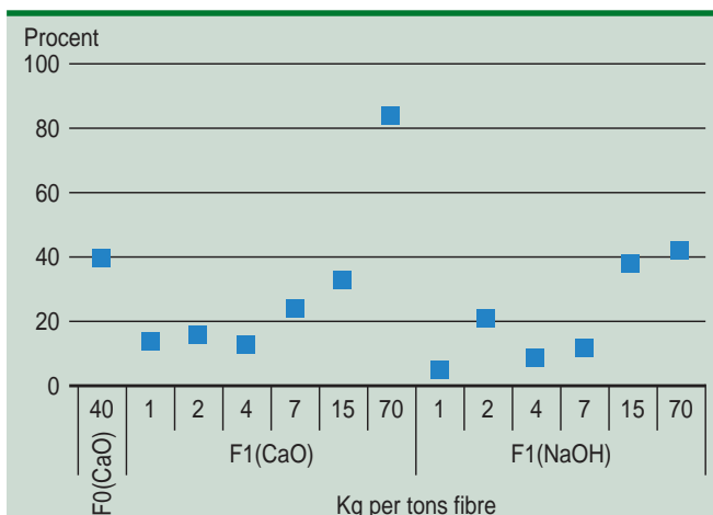
Figur 2: Merudbytte i procent ved varierende mængder brændt kalk (CaO) og NaOH i kg/ton. F0 er fibre fra biogasfællesanlæg i Fangel, mens F1 er fibre fra gårdanlæg i Præstø.
