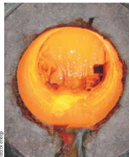
Til højre: Et kig ind i reaktoren på forsøgsanlægget, der blev brugt til forgasning af spildevandsslam. Læg mærke til, hvordan slaggen sætter sig på væggen og løber ud i bunden af reaktoren.
