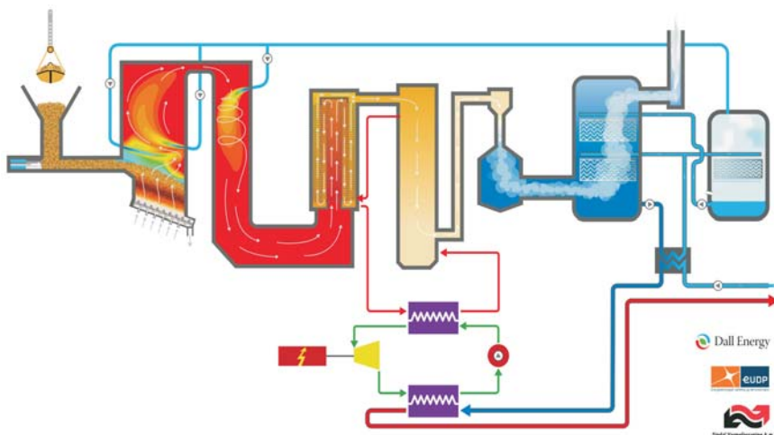
Figur 1. Biomasse føres med kran fra brændselslageret til indføderen, som skubber biomassen ind i forgasseren, hvor biomassen omdannes til gas. Gassen afbrændes i to trin, hvorefter røggassen afgiver sin energi til termoolie-systemet. Termoolien driver ORC-turbinen, som producerer el og varme. Restenergien fra røggassen udnyttes til fjernvarme i røggasskrubberen.
